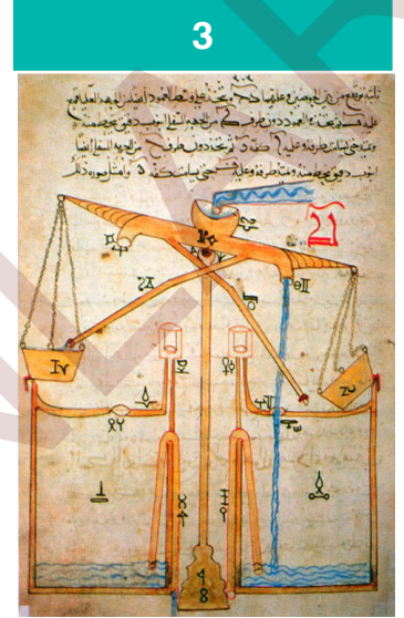
Su gücü ile çalışan bir kaldırma makinesi çizimi
